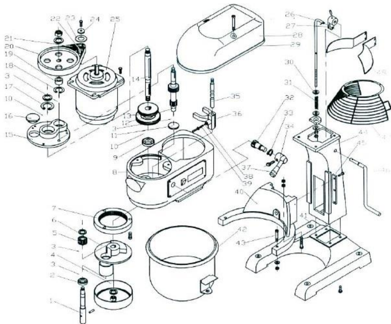
Рис 8. Основные элементы для модели В-20ФА
